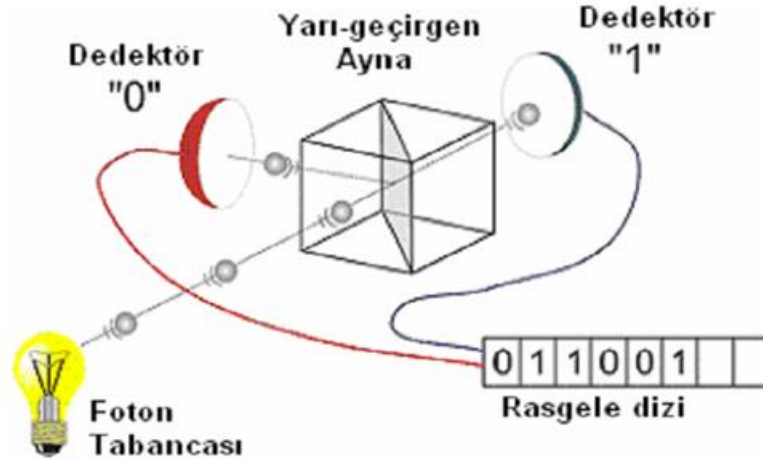
Şekil 3 Kuantum Rastgele Sayı Üretici
