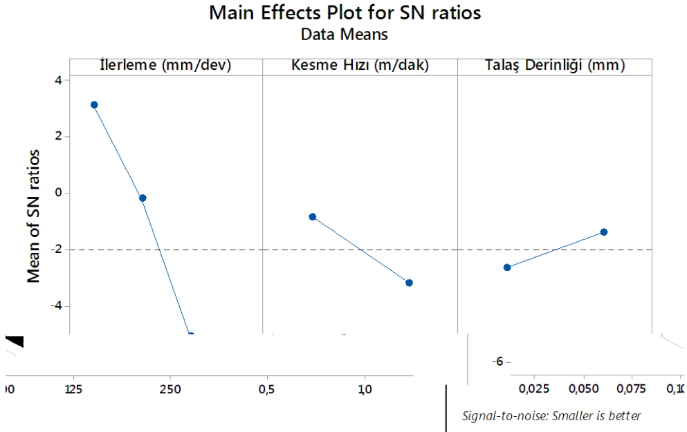
Şekil 5. Faktörlerin Bireysel Etkileri (S/N Oranları)
